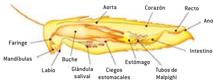
Aparato digestivo, circulatorio y excretor de los artrópodos.
