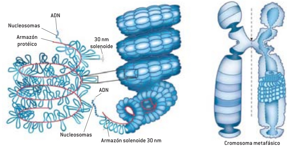
Estructura del cromosoma y del ADN que lo conforma.
