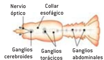
Sistema nervioso ganglionar de los artrópodos
