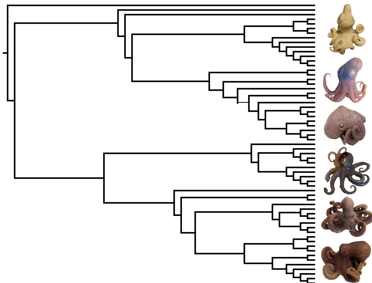
Figura 3. Arbol de especies que contiene información sobre los patrones (topología) de la diversificación de especies.
