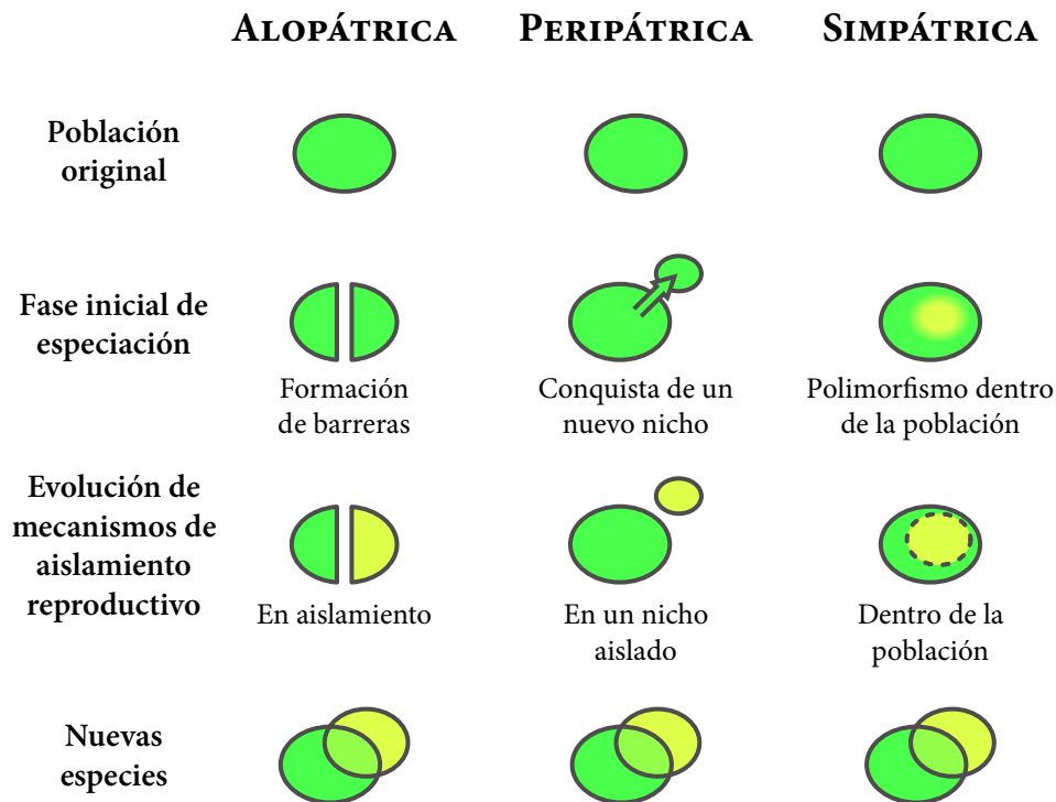
Figura 4. Esquema de tres modelos de especiación donde se enfatiza en forma comparativa cuatro etapas en el proceso de especiación.
